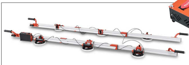
Power-Vacuum kit montato su EASY-MOVE mkiv senza traverse (Art. 432HAKITR + Art. 432EM04CA).
