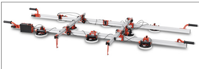
Power-Vacuum kit montato su EASY-MOVE mkiv con traverse (Art. 432HAKITR + Art. 432EM04TA).
